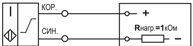
Схема подключения к оборудованию
