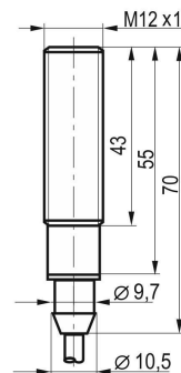
Габаритный чертеж
